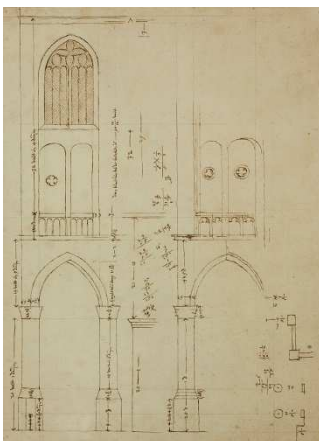
Opmetingen van de muren van het schip en het transept van de Grote of Sint-Laurenskerk te Alkmaar ongedateerd (1661?)
